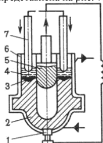
Рис.7.3. Схема изготовления отливок электрошлаковым литьем
