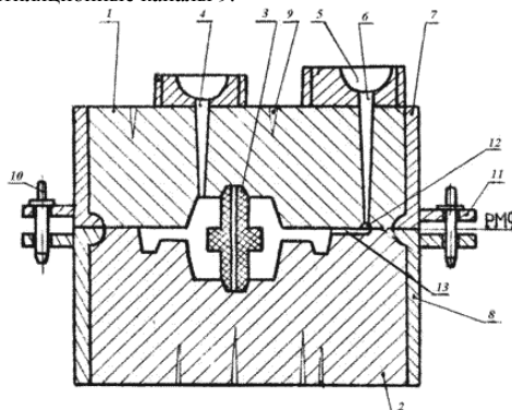
Рис. 5.2. Литейная форма
