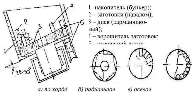
Рис. 3.21. Схема дискового карманчатого бункера
