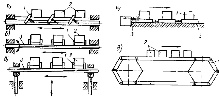
Рис. 4.4. Схемы транспортеров автоматических линий с жёсткой связью:
