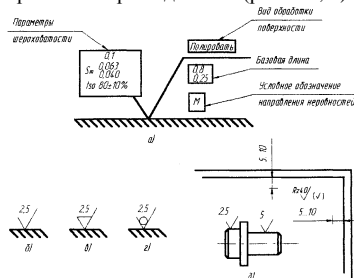
Рис. 6.6. Структура обозначения шероховатости поверхности
