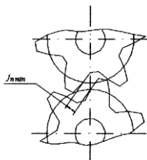
Рис. 6.10. Боковой зазор J_n в зубчатой передаче
