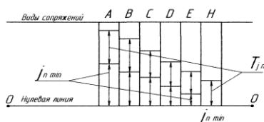
Рис. 6.11. Виды сопряжений и допуски на боковой зазор в зубчатых передачах
