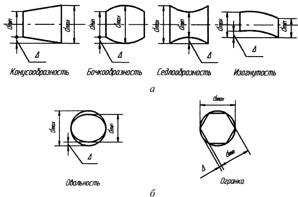
Рис. 6.4. Отклонения формы цилиндрических поверхностей: в продольном ( a ) и поперечном ( б ) сечениях
