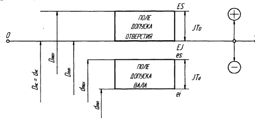
Рис. 6.2. Поля допусков отверстия и вала
