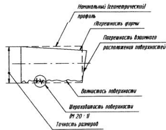
Рис. 6.3. Составляющие геометрической точности деталей (вала)
