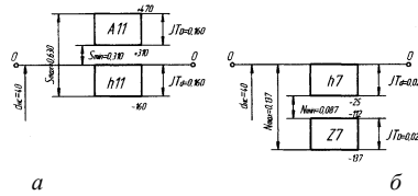
Рис. 6.8. Обозначение посадок в системе вала
