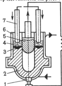
Рис.7.3. Схема изготовления отливок электрошлаковым литьем
