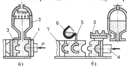
Рис. 5.6. Изготовление безопасных литейных форм
