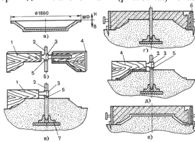
Рис.5.4. Шаблонная формовка
