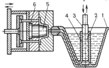
Рис.7.2. Схема изготовления отливки на машинах с горячей камерой прессования
