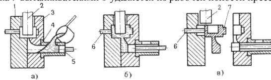
Рис.7.1. Технологические операции изготовления отливок на машинах с горизонтальной холодной камерой прессования
