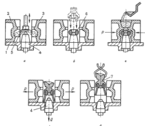
Рис. 6.3 Технологические операции изготовления отливки в кокиль
