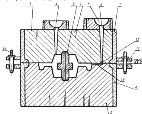
Рис. 5.2. Литейная форма
