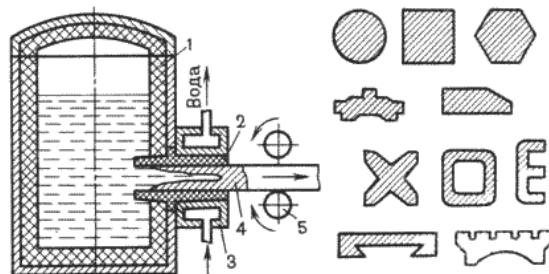
Рис. 7.4. Схема непрерывного литья (а) и разновидности получаемых отливок (б) Разливка стали
