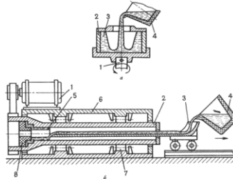
Рис.6.4. Схемы процессов изготовления отливок центробежным литьем
