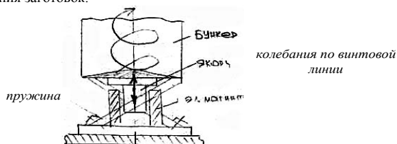
Рис. 3.26. Схема вибробункера с тангенциальными вибраторами
