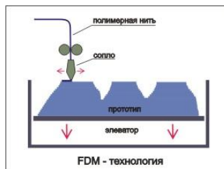
Рис. 5.6. Принцип работы FDM-машины
