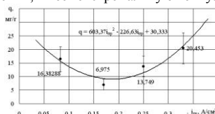
Зависимость удельного расхода от плотности тока правки: V = 35 \text{ м/с} ; S = 1,5 \text{ м/мин} ; t = 0,02 \text{ мм/дв.ход} ; i_{np} = 6,25 \text{ A/cm}^2 ; - Р6М5; АС6 80/63 А1 4 М1
