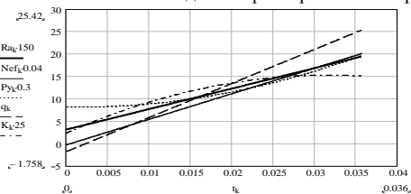
Графическая зависимость выходных параметров от глубины резания
