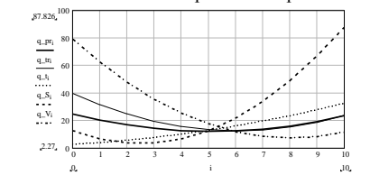
Графическая зависимость удельного расхода шлифовального круга от режимов обработки
