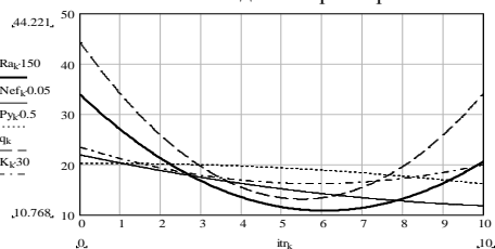
Графическая зависимость выходных параметров от тока травления
