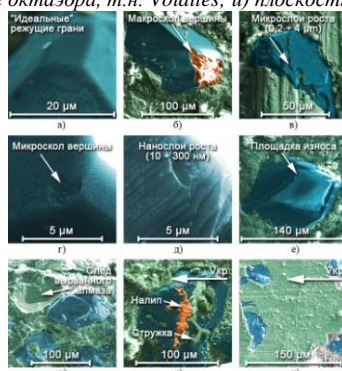
Рис. 4. Кристаллы алмаза с характерными для шлифования видами износа (разрушения режущих граней): а) режущая грань алмаза до шлифования; б) объемное разрушение вершины алмаза в виде макроскола; в) износ режущей поверхности алмаза по микрослоям роста; г) объемное разрушение вершины алмаза в виде микроскола; д) износ режущей поверхности алмаза по нанослоям роста; е) истирание режущей поверхности алмаза с образованием гладкой площадки износа; ж) вырывание алмаза из связки шлифовального круга; з) образование налива на режущей грани алмаза; и) алмазы, полностью покрытые засаленным слоем
