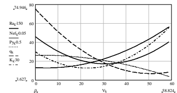
Графическая зависимость выходных параметров от скорости резания
