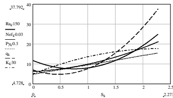
Графическая зависимость выходных параметров от продольной подачи
