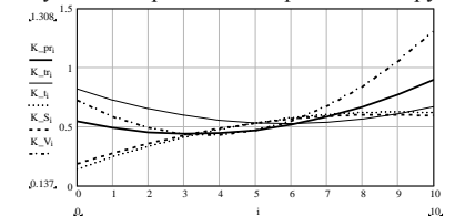
Графическая зависимость коэффициента режущей способности от режимов обработки
