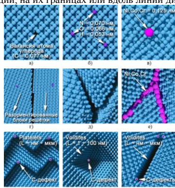
Рис. 3. Моделируемые дефекты синтетического алмаза, с учетом внутренней морфологии кристалла. Точечные дефекты (микродефекты): а) вакансии; б) замещенные атомы (С-дефект); в) межузельные атомы; г) дислокации. Объемные дефекты (макродефекты): д) трещины между блоками; е) металлические включения; ж) пластинчатые дефекты, т.н. Platelets; з) субмикроразрывы в форме октаэдра, т.н. Voidites; и) плоскостные субмикроразрывы
