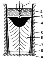
Рис.3.5. Схема электрошлакового переплава
