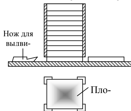
Рис. 3.3. Схема шахтного магазина
