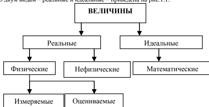
Рис. 1.1. Классификация величин
