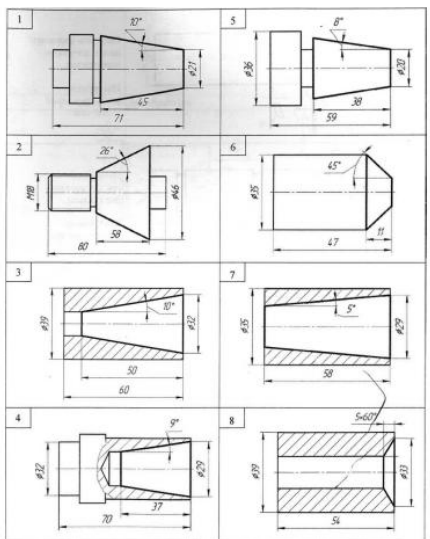
Рис. 1. Эскизы деталей для обработки конической поверхности
