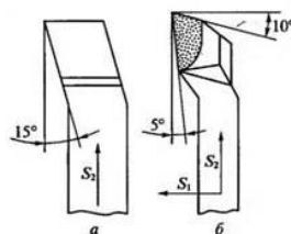
Рис. 6.11. Подрезной резец: а – из быстрорежущей стали; б – армированный пластинкой твердого сплава; S_1 и S_2 – подача
