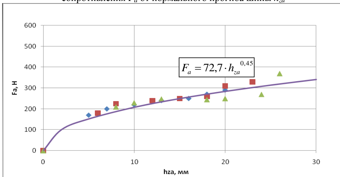
Диаграмма зависимости амплитудных значений силы неупругого сопротивления F_a от нормального прогиба шины h_{za}
