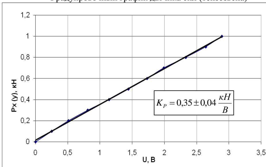
Градуировочный график датчика сил (тензозвена)
