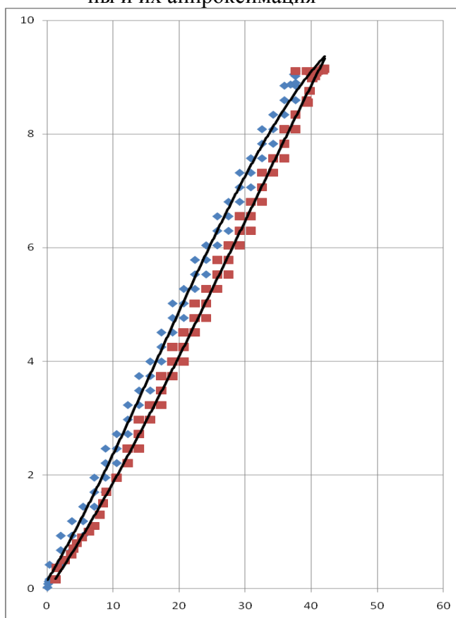
Диаграммы с экспериментальными характеристиками нормальной жесткости шины 7.35-14 ИД-195 при различных значениях внутреннего давления воздуха для случая бокового догружения колеса
