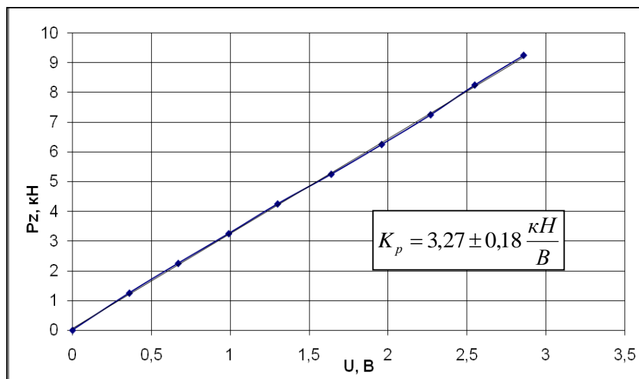
Градуировочный график датчика сил (тензооси)
