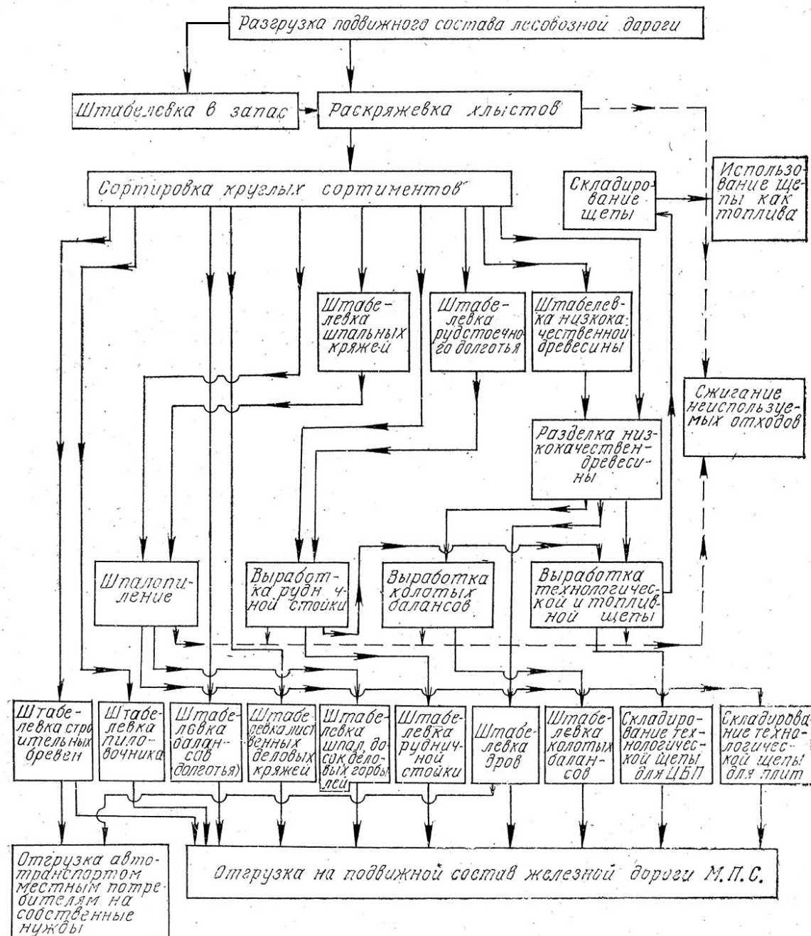
Рисунок - Структурная схема технологического процесса лесопромышленного склада
