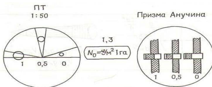
Рис. 8 Смещение рассматриваемой части ствола при работе с призмой
