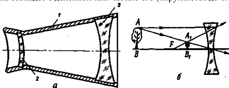
Рис.5 - Оптический высотомер Н.П.Анучина а - устройство прибора; б - схема образования изображения:
