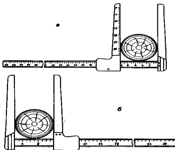
Рис. 1 - Деревянная мерная вилка: а - сторона с 2-сантиметровой шкалой; б - сторона с 4-сантиметровой шкалой
