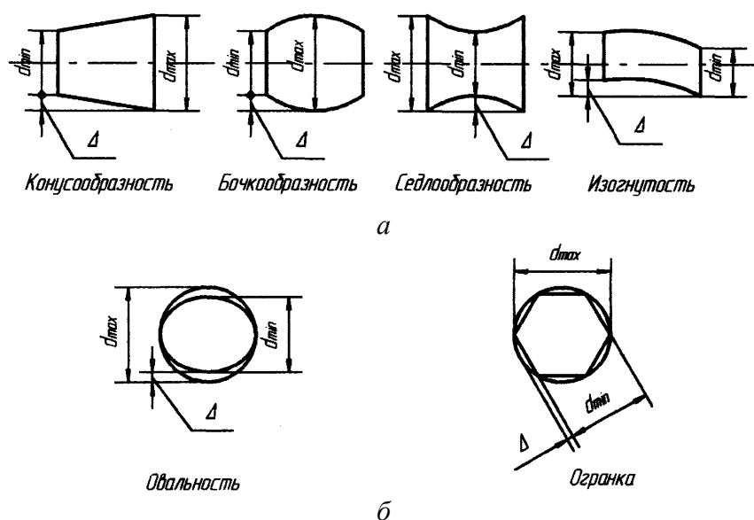
Рис. 6.4. Отклонения формы цилиндрических поверхностей: в продольном ( a ) и поперечном ( б ) сечениях
