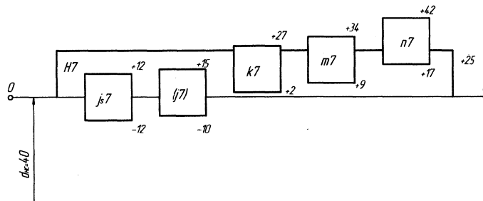
Рис. 6.9. Схема полей допусков переходных посадок: ( j7 ) – дополнительное поле допуска вала ограниченного применения
