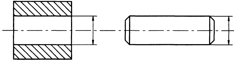
Рис. 6.10. Обозначение предельных отклонения линейных размеров деталей: а – \varnothing 40H8 , \varnothing 40e8 ; б – \varnothing 40 \begin{pmatrix} +0,039 \\ -0,089 \end{pmatrix} , \varnothing 40 \begin{pmatrix} -0,050 \\ -0,089 \end{pmatrix} ; в – \varnothing 40H8 \begin{pmatrix} +0,039 \\ -0,089 \end{pmatrix} , \varnothing 40e8 \begin{pmatrix} -0,050 \\ -0,089 \end{pmatrix}
