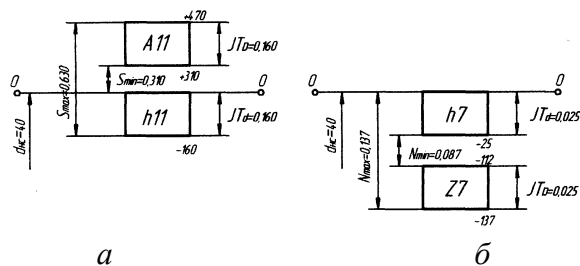
Рис. 6.8. Обозначение посадок в системе вала и их схемы полей допусков: а – с зазором S
