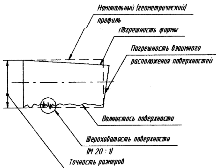
Рис. 6.3. Составляющие геометрической точности деталей (вала)
