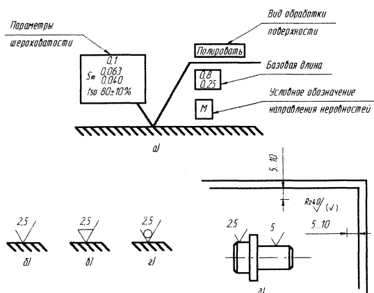
Рис. 6.6. Структура обозначения шероховатости поверхности
