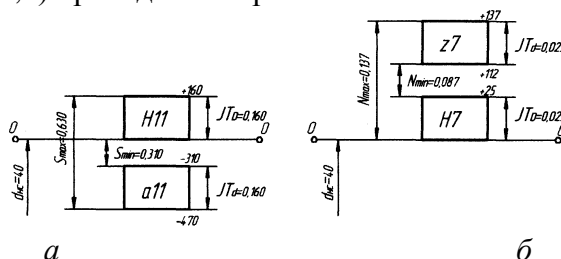
Рис. 6.7. Обозначение посадок в системе отверстия и их схемы полей допусков:
