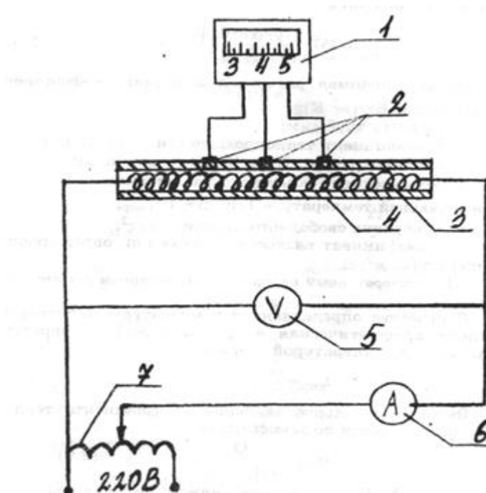
1 - измерительный прибор, 2 - термодатчик, 3 - электронагреватель, 4 - латунная трубка, 5- вольтметр, 6 - амперметр, 7 – автотрансформатор
