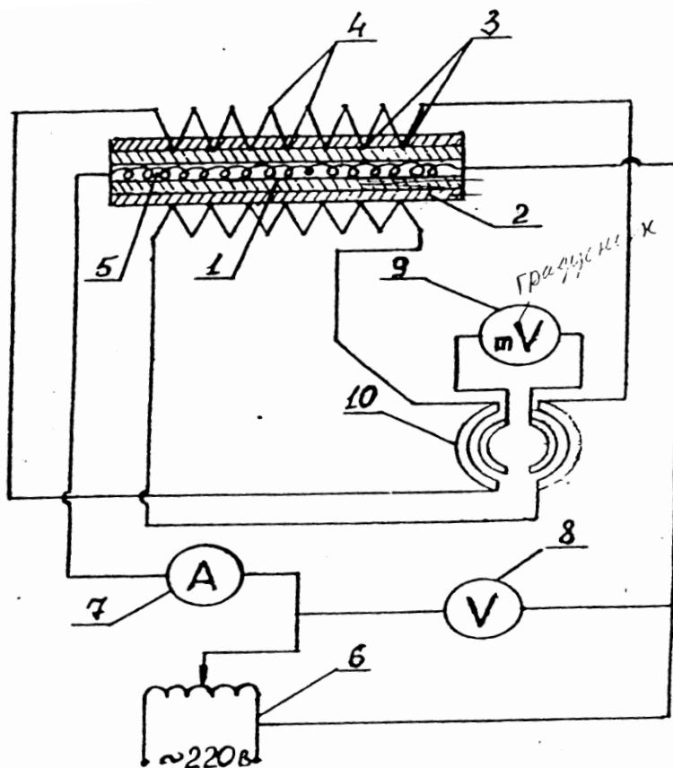
Рис. 1.1 Схема установки: 1 - латунная трубка, 2 - слой теплоизоляции, 3-горячие спай термопар, 4-холодные спай термопар, 5 - электронагреватель, 6 - автотрансформатор, 7 - амперметр, 8 - вольтметр, 9 - милливольтметр, 10 - переключатель термопар
